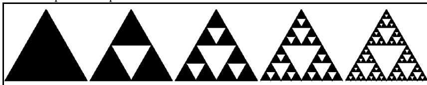
Рисунок 1 – Построение треугольника Серпинского
